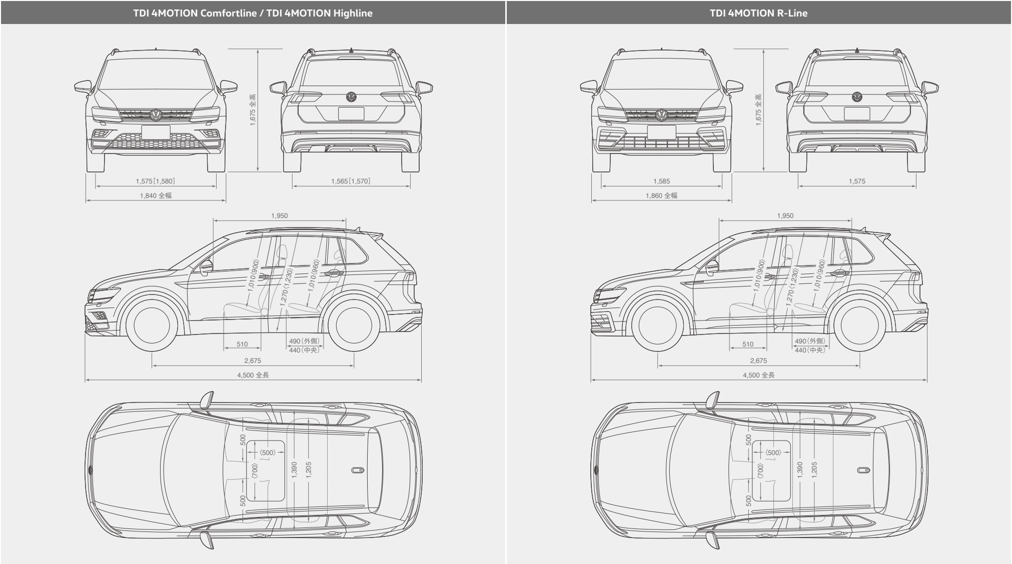
四面図(mm)
